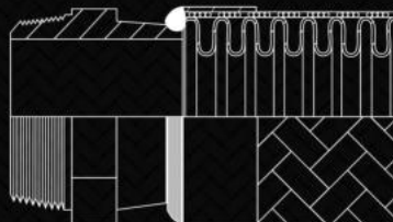
Fixed male – Maschio fisso
