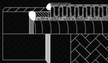
Protezione interna con tubo a doppia aggraffatura
