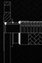
Fixed flange "A" – Flangia fissa "A"
