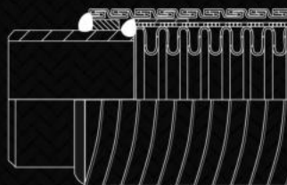
Protezione esterna con tubo a doppia aggraffatura
