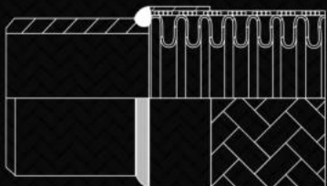
Welding end – Manicotto liscio a saldare
