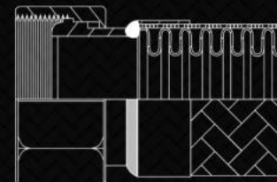
Swivel female cone seat – Femmina girevole sede ogiva
