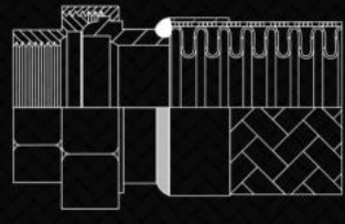
Union Coupling – Bocchettone a tre pezzi
