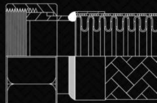
Swivel female flat seat – Femmina girevole sede piana
